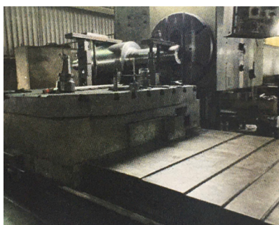
Máy doa ngang
