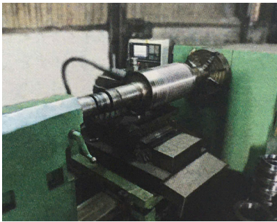
Máy phay rãnh vằn
