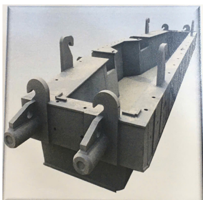
Thùng rót thép trung gian
