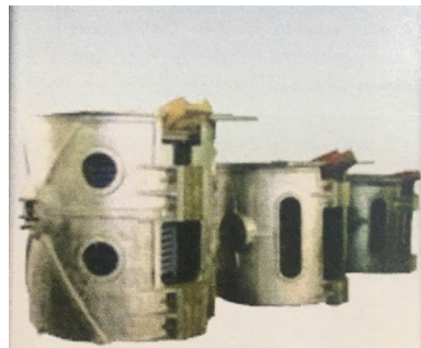
Lò trung tần
