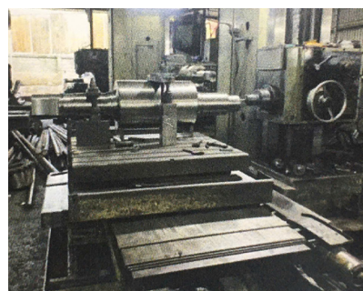
Máy doa ngang
