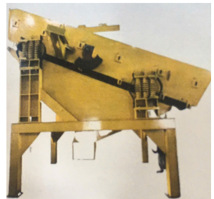
Sàn rung liệu
